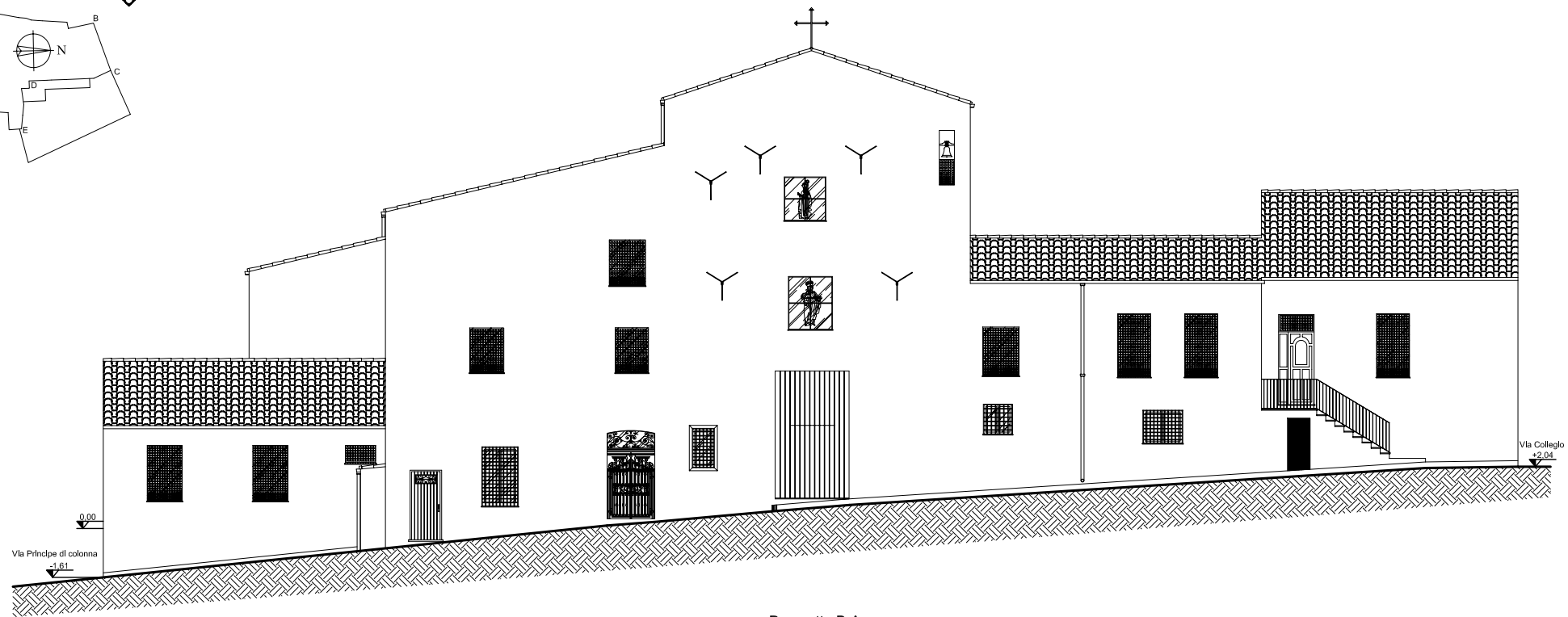
Prospetto B-A Scala 1:100
